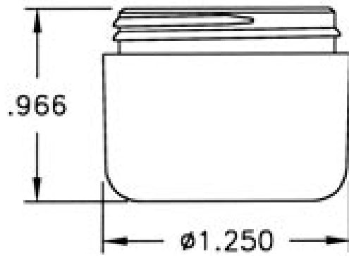
1/4oz. 3025
